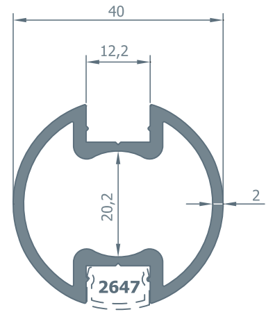
2839 0.870 kg/m
