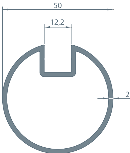
221 0.943 kg/m
