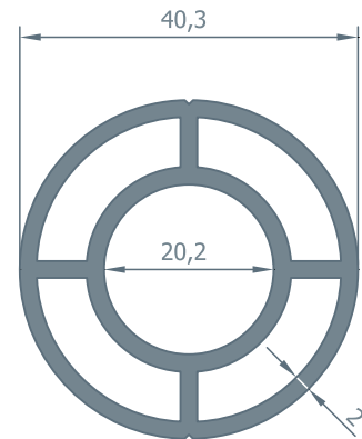
5955 1.179 kg/m
