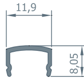
2647 0.068 kg/m
