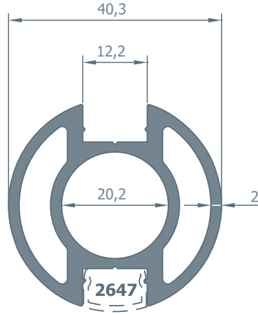
2646 1.165 kg/m
