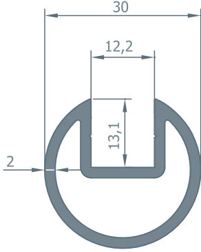
204.26 0.607 kg/m
